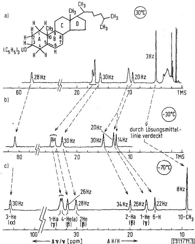
Abbild. 5. ^1H -NMR-Spektren des Cholesteryl-Teils (Ringe A und B) der Verbindung (C_5H_5)_3UOC_{27}H_{45} ( 3 ) bei variabler Temperatur; Meßfrequenz 90 MHz; Lösungsmittel Toluol- d_8 ; interner Standard C_6H_5 -Linie des Lösungsmittels, als Nullpunkt der Abszissenskala wurde der besseren Übersicht wegen die Lage der TMS-Resonanz gewählt
