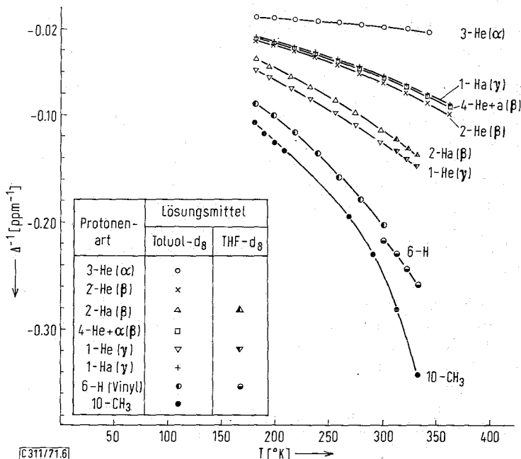
Abbild. 6. 1/\Delta -gegen- T -Diagramme der paramagnetischen Verschiebungen \Delta einiger Cholesterin-Linien im ^1\text{H} -NMR-Spektrum von (\text{C}_5\text{H}_5)_3\text{UOC}_{27}\text{H}_{45} ( 3 )
