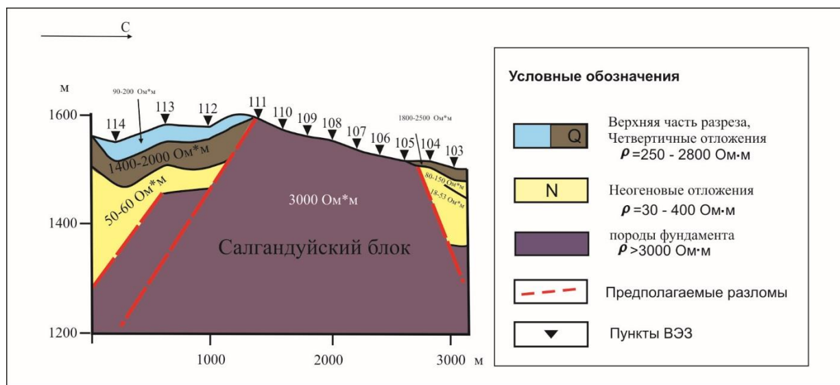
Рис. 3. Модель Салгандуйского блока с учетом результатов трехмерного моделирования
