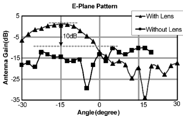
Fig. 25. E-plane antenna gain.
