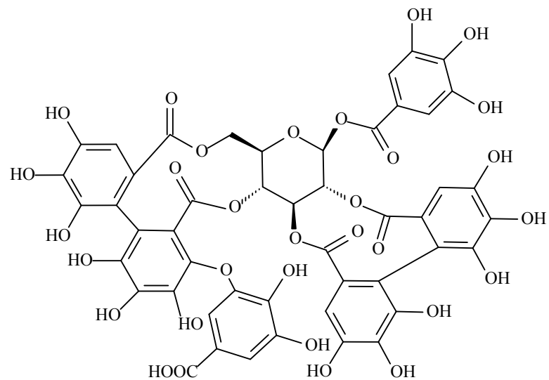
24a rubusuaviin A
