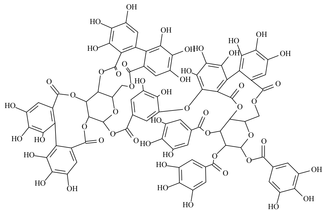
24b rubusuaviin B
