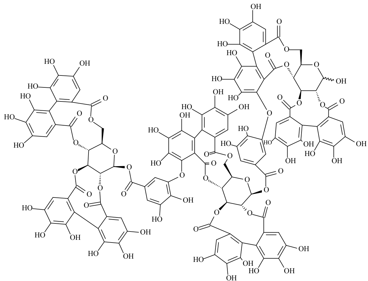
24d rubusuaviin D
