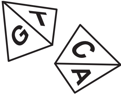
Fig. 1. DNA dice.
