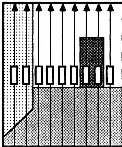
linear sampling
