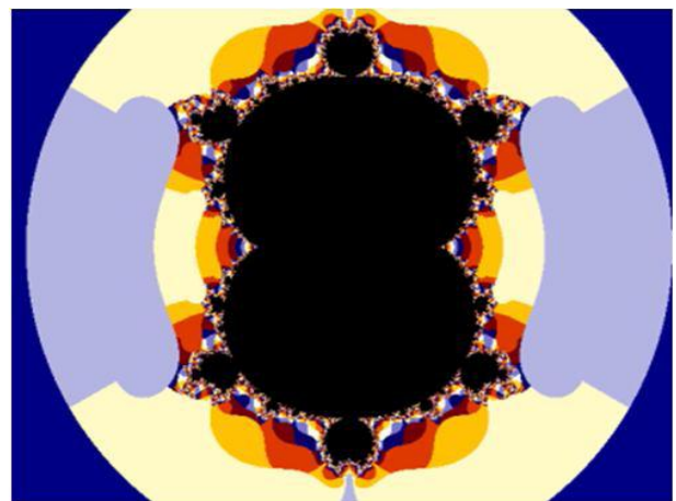
Fig.7 : Relative Superior Mandelbrot Set for s= s'=1
