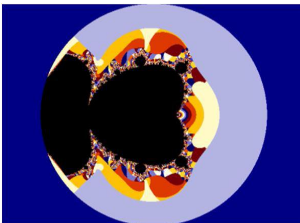
Fig.5 : Relative Superior Mandelbrot Set for s= s'=1
