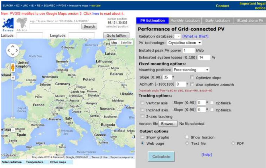
Fig. 1 PVGIS Interface
