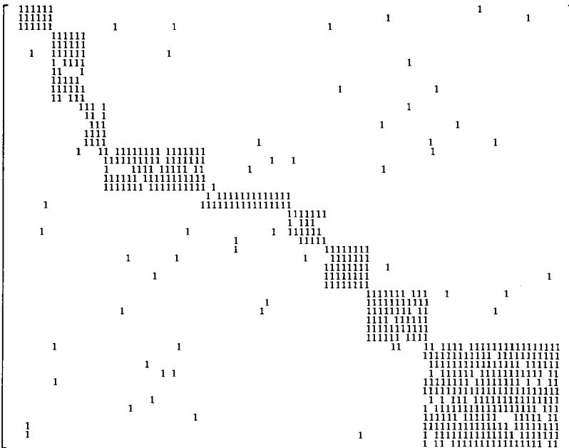
(d) Clumpiness = 9
