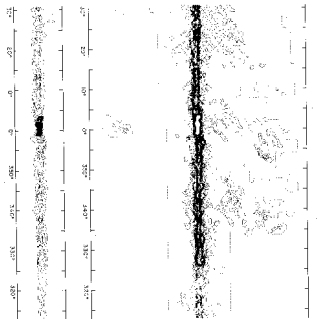
Galactic Latitude vs. Galactic Longitude
