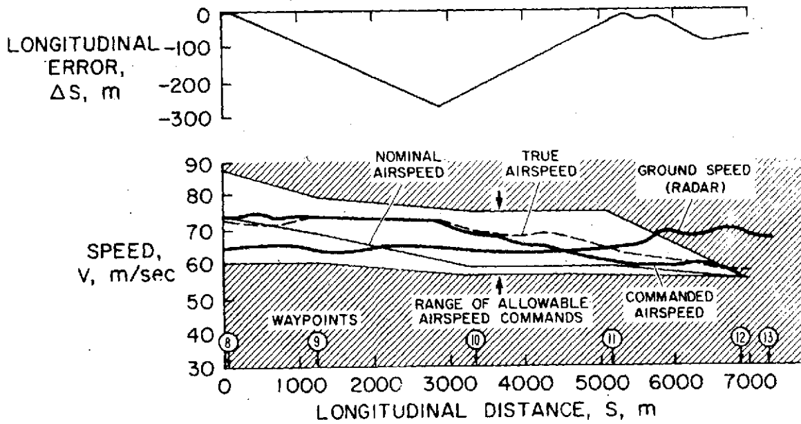
Figure 10.- Longitudinal guidance.
