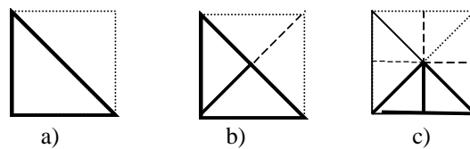
FIGURE 2. Bitree subdivision
