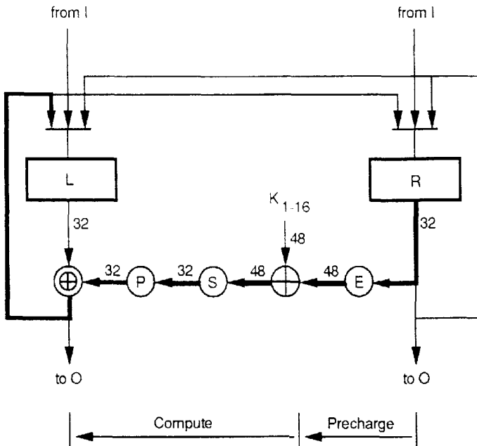
Fig. 9. One DES Iteration
