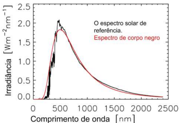
Figura 1: O espectro solar de referência em condições de baixa atividade solar (linha preta ou linha que apresenta variações) [14] e o espectro solar como se o Sol fosse um corpo negro com uma temperatura de \sim 5.800 K (linha vermelha ou contínua), adaptado de [13].
