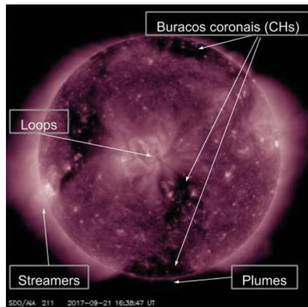
Figura 6: Fenômenos na coroa solar: Linhas de campo fechadas (loops), buracos coronais (CHs), Helmet streamers , plumes nos polos do Sol. Adaptado da imagem do instrumento AIA no comprimento de onda 21,1 nm, no dia 21 de setembro de 2017.
