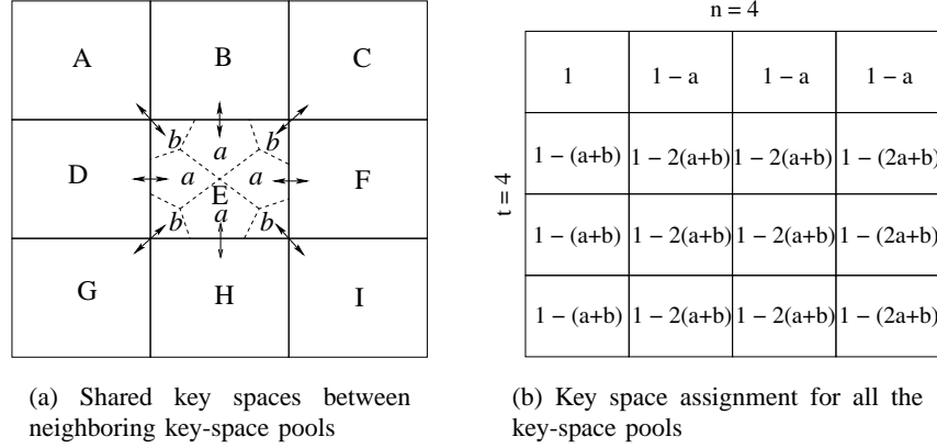
Fig. 3. Key-Space Pools
