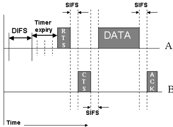
802.11 DCF MAC
