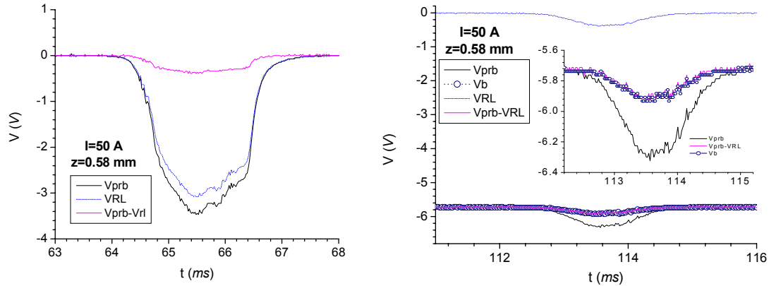
Figure 8.14 I=50 A, probe N.12, z=0.58 mm.
