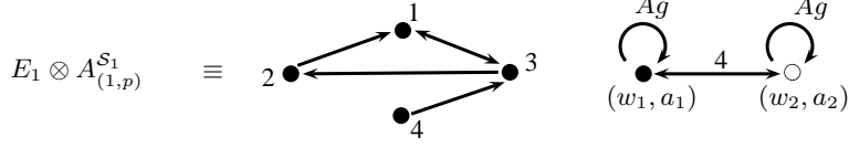
Fig. 5. Example Update Result.
