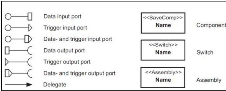
Fig. 5. The graphical notation of SaveCCM
