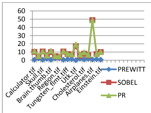
PSNR
