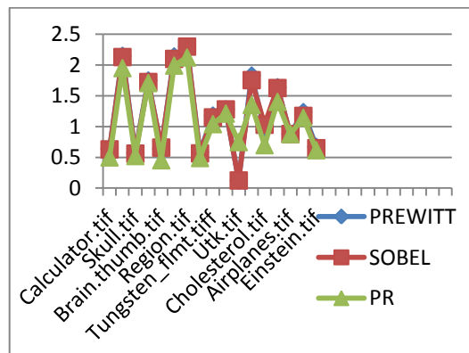
MSE
