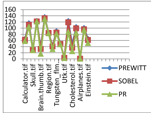
AD
