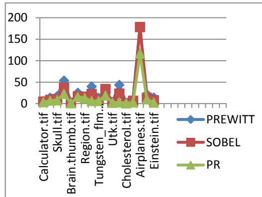
SC
