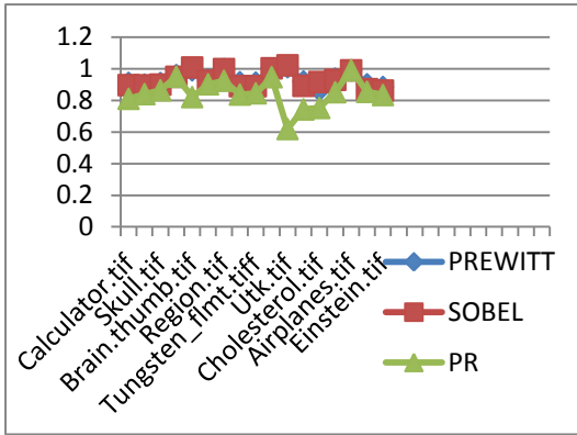
NAE
