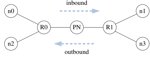
Fig. 8. A Tmix topology
