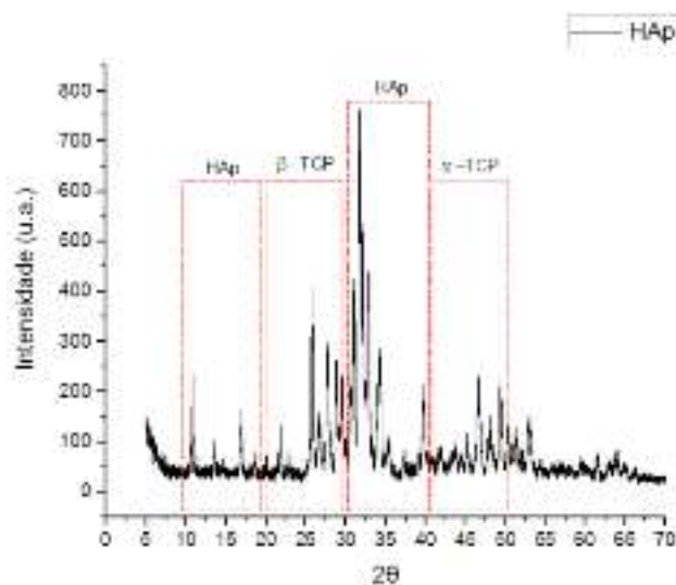
Figura 2: DRX do pó da HAp.
