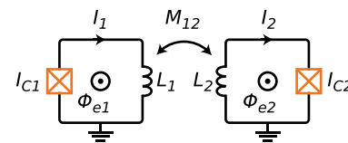
(d) Inductive coupling via coupler
