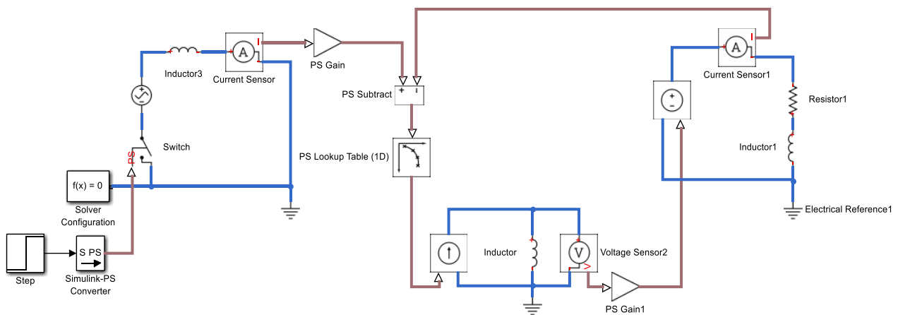
Рис. 3. Модель трансформатора тока в среде MATLAB Simscape Fig. 3. Model of a current transformer in MATLAB Simscape environment
