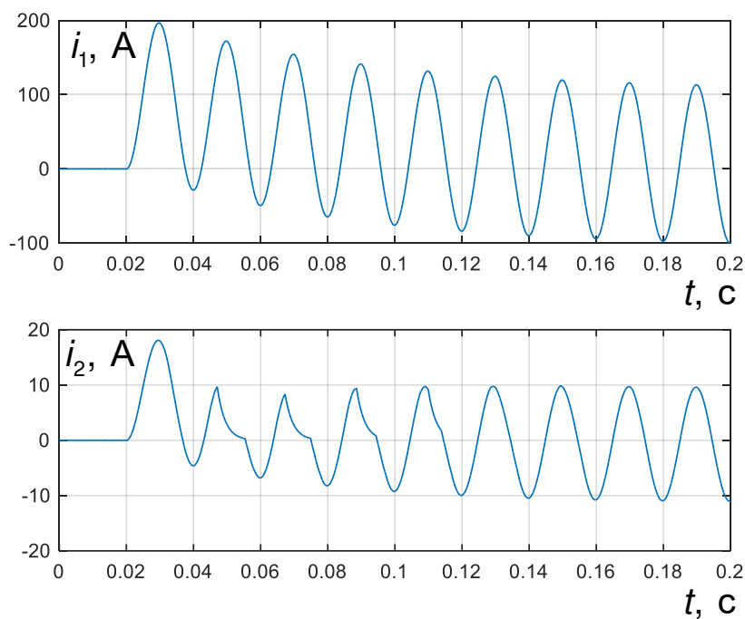
Рис. 8. Осциллограммы токов в первичной и вторичной обмотках трансформатора тока в переходном режиме с аperiodической составляющей тока при первичном токе 75 А и вторичной нагрузке R_2 = 0,96 Ом, L_2 = 2,292 мГн Fig. 8. Oscillograms of currents in primary and secondary windings of the current transformer in the transient mode with an aperiodic current component at a primary current of 75 A and a secondary load R_2 = 0.96 Ohm, L_2 = 2.292 mH
