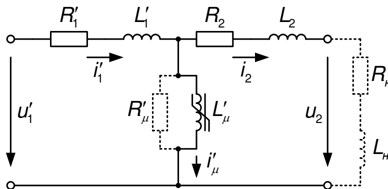
Рис. 1. Т-образная схема замещения трансформатора тока Fig. 1. T-shaped equivalent circuit of a current transformer
