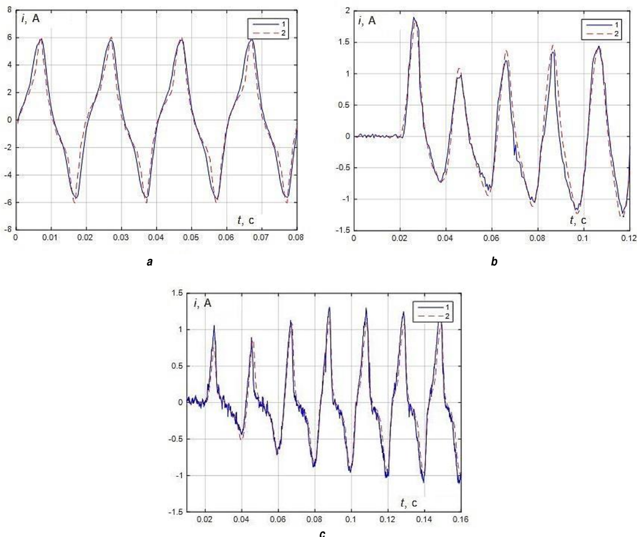
Рис. 10. Осциллограммы вторичного тока при первичном токе 50 А в установившемся режиме и вторичной нагрузке 9,6 Ом (а), при первичном токе 10 А с аperiodической составляющей и вторичной нагрузке 9,6 Ом (b) и при первичном токе 10 А с аperiodической составляющей и вторичной нагрузке 39 Ом (с): 1 – расчетные осциллограммы в MATLAB Simulink; 2 – осциллограммы, записанные осциллографом Fluke 190 Fig. 10. Oscillograms of the secondary current at a primary current of 50 A in the steady state and a secondary load of 9.6 Ohm (a), at a primary current of 10 A with an aperiodic component and a secondary load of 9.6 Ohm (b) and at a primary current of 10 A with an aperiodic component and a secondary load of 39 Ohm (c): 1 – calculated oscillograms in MATLAB Simulink, 2 – oscillograms recorded by a Fluke 190 oscilloscope
