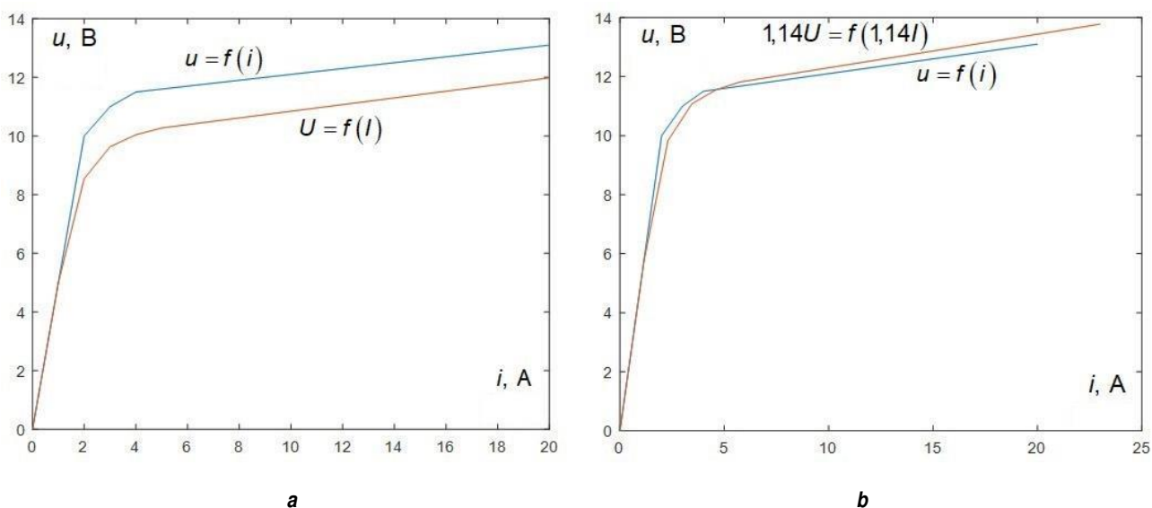
Рис. 5. Вольтамперные характеристики нелинейного сопротивления, снятые в мгновенных и действующих значениях (а), и те же характеристики после умножения вольтамперной характеристики в действующих значениях на коэффициент 1,14 по току и напряжению (b) Fig. 5. Current-voltage characteristics of nonlinear resistance taken in instantaneous and effective values (a), the same characteristics after multiplication of the current-voltage characteristic in effective values by a factor of 1.14 for current and voltage (b)
