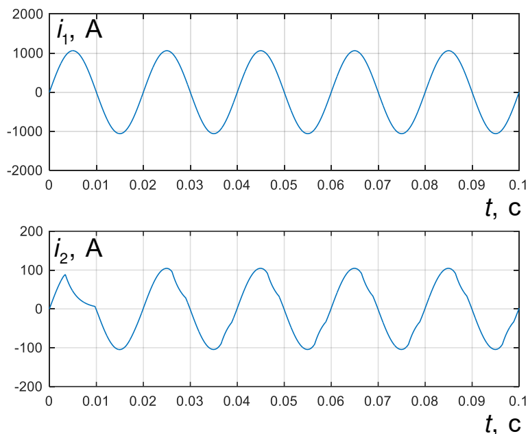
Рис. 7. Осциллограммы токов в первичной и вторичной обмотках трансформатора тока при первичном токе 750 А и вторичной нагрузке R_2 = 0,48 Ом, L_2 = 1,146 мГн Fig. 7. Oscillograms of currents in primary and secondary windings of the current transformer at a primary current of 750 A and a secondary load R_2 = 0.48 Ohm, L_2 = 1.146 mH
