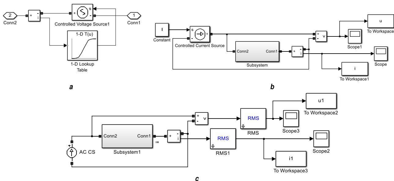
Рис. 4. Модель нелинейного сопротивления (а), получение вольтамперной характеристики в мгновенных значениях (b) и в действующих значениях (c) Fig. 4. Model of nonlinear resistance (a), obtaining of current-voltage characteristics in instantaneous (b) and effective values (c)
