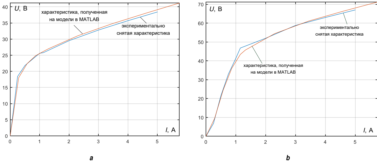
Рис. 9. Сравнение экспериментально снятой и полученной на модели вольтамперных характеристик трансформатора тока типа ТПЛ-10 50/5 (а) и ТВЛМ-10 75/5 (б)
