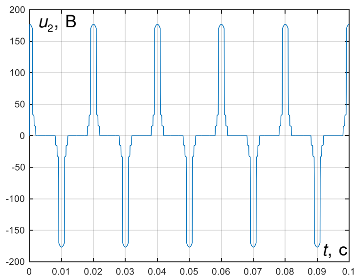
Рис. 6. Осциллограмма напряжения на вторичной обмотке трансформатора тока при разомкнутой вторичной обмотке и первичном токе 50 А
