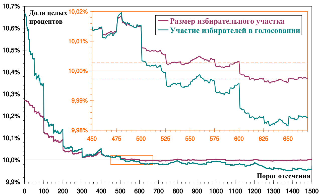
Рис. 3. Эмпирическая вероятность получения целых процентов
