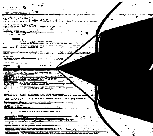
(d) Configuration 1.278-29.82-44.2 o ; \alpha = +1/2^{\circ}
