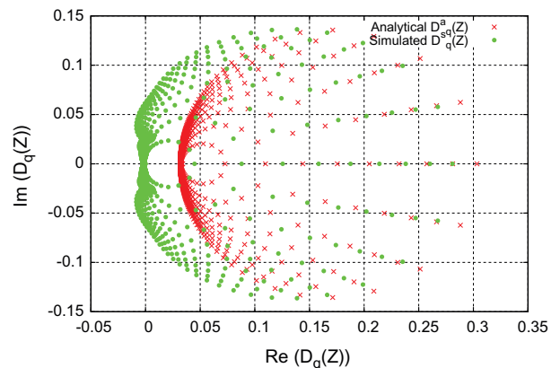
(b) M/M/1
