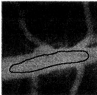
(d) Initialization 2
