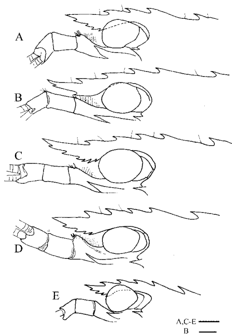
Figure 2. Rostral variation within Lysmata wurdemanni (Gibbes 1850). (A) USNM 1082794. (B) USNM 1082798 Neotype. (C) USNM 1082793. (D) USNM 77754. (E) USNM 1082794. Scales A–E 1 mm.
