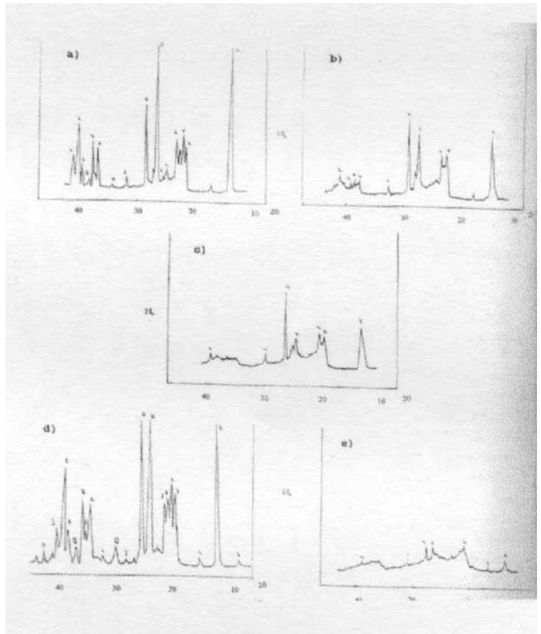
Figura 2. Difractogramas de las muestras. Caolín TR molido a) Crudo b) Molido 5 min c) Molido 10 min d) Micronizado 16 horas e) Molido 10 min secado 300°C
