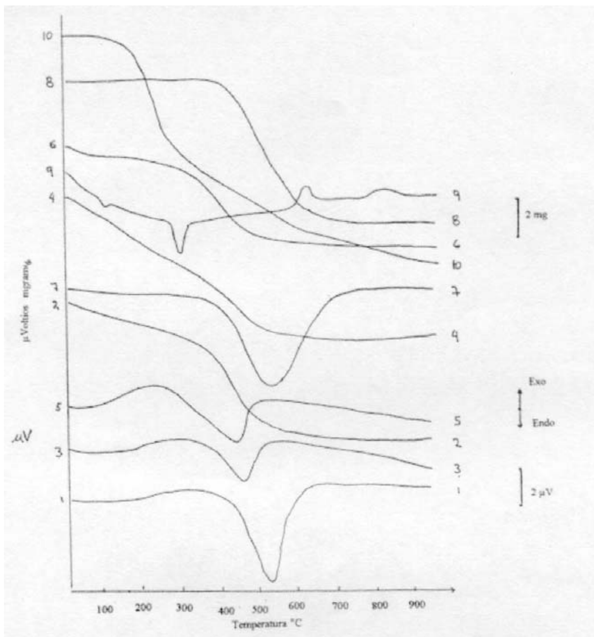
Figura 3. Curvas de calentamiento. Análisis termogravimétrico. Activación mecánica del caolín IG 1) DTA Crudo 2) TGA Crudo 3) DTA Calcinado 4) TGA Calcinado 5) DTA Molido 5 min 6) TGA Molido 5 min 7) DTA Molido 10 min 8) TGA Molido 10 min
