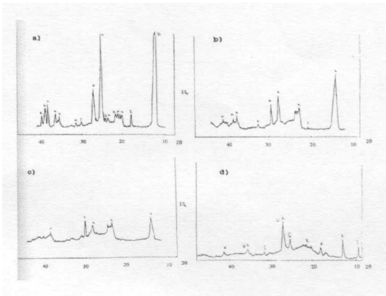
Figura 1. Difractogramas de las muestras. Caolín IG molido a) Crudo b) Molido 5 min c) Molido 10 min d) Calcinado
