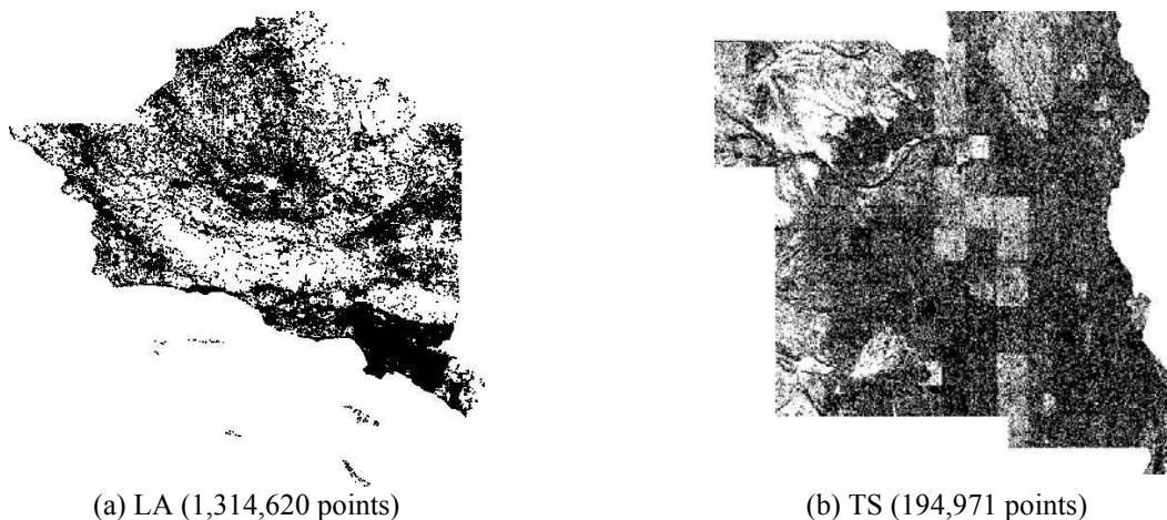
Fig. 29. Real datasets
