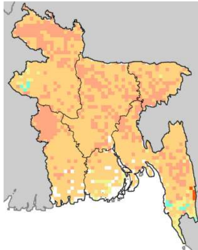
d. MIROC
