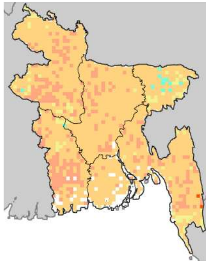
d. MIROC
