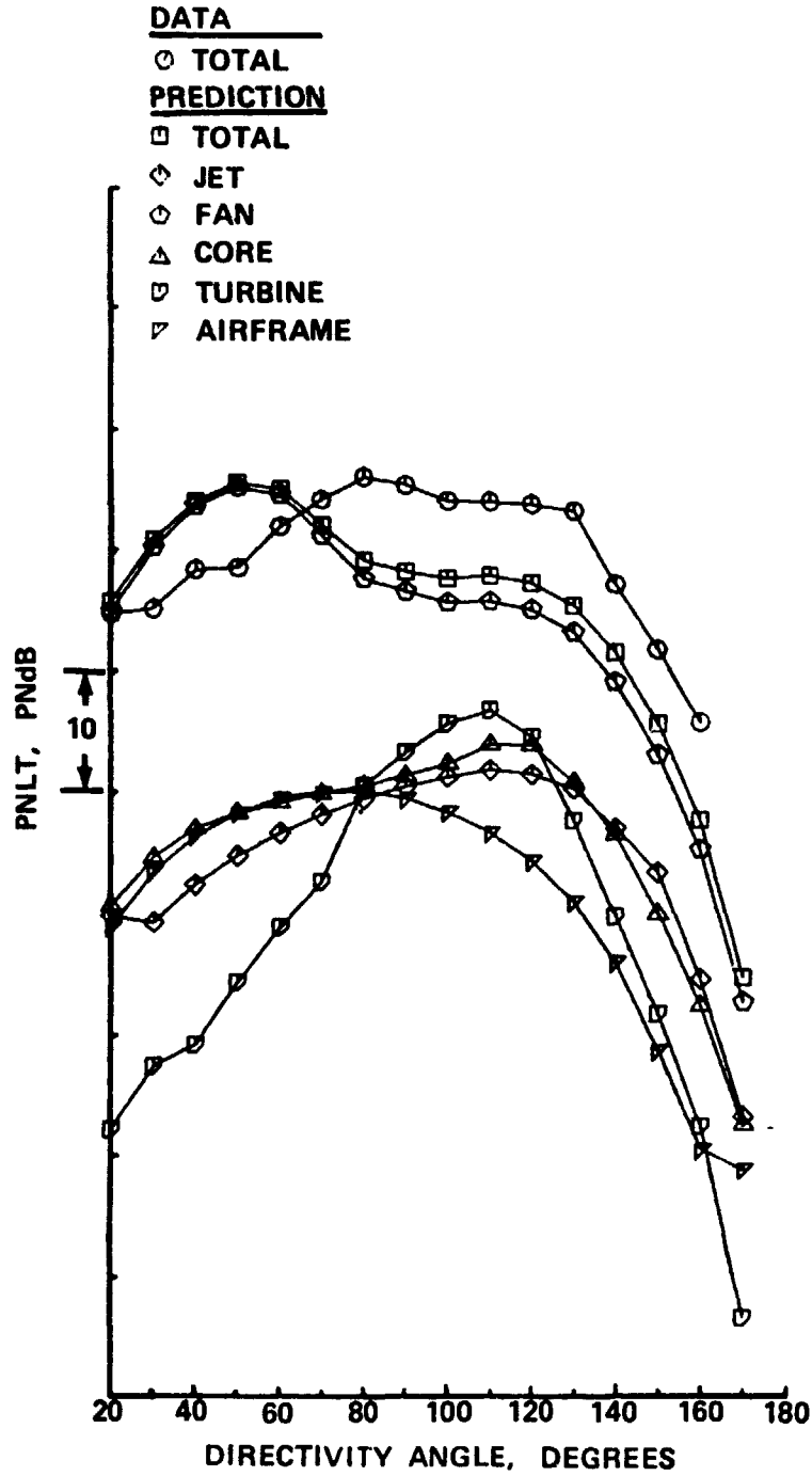
(d) ENGINE POWER SETTING, % N1C = 89.5
