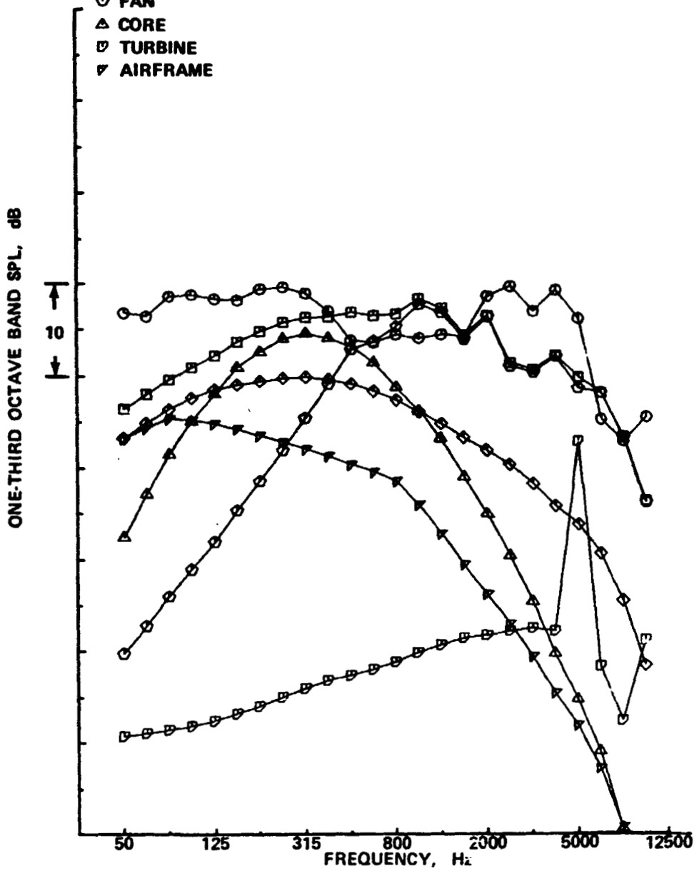
(d) DIRECTIVITY ANGLE = 120°
