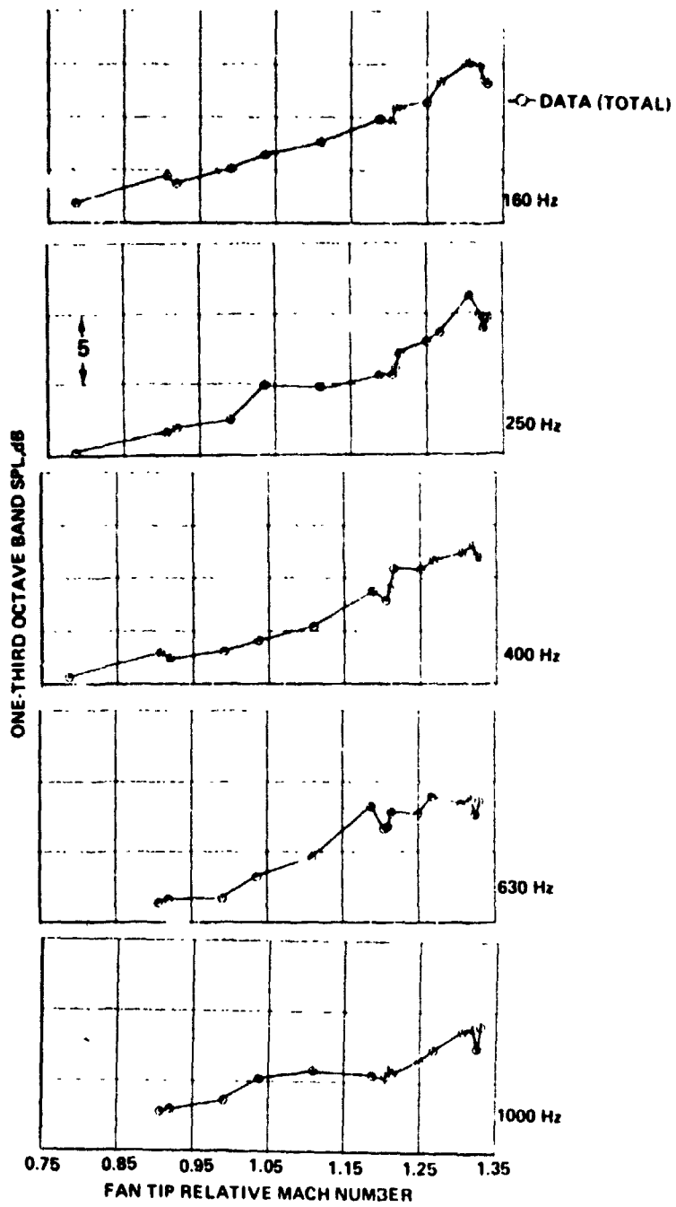
(d) DIRECTIVITY ANGLE 120°
