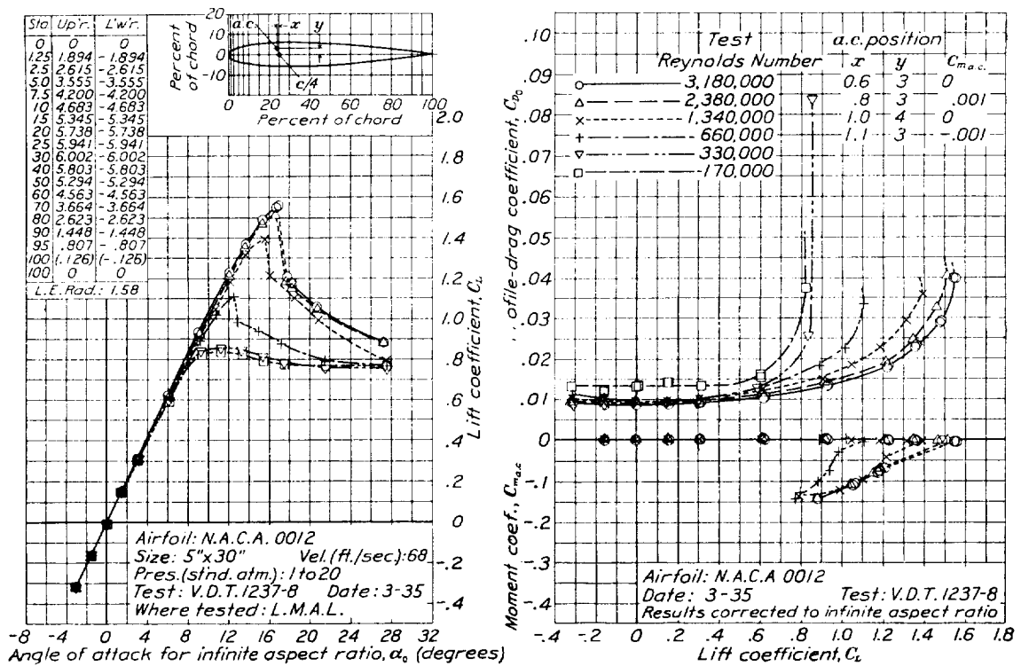
FIGURE 3.—N. A. C. A. 0012.
