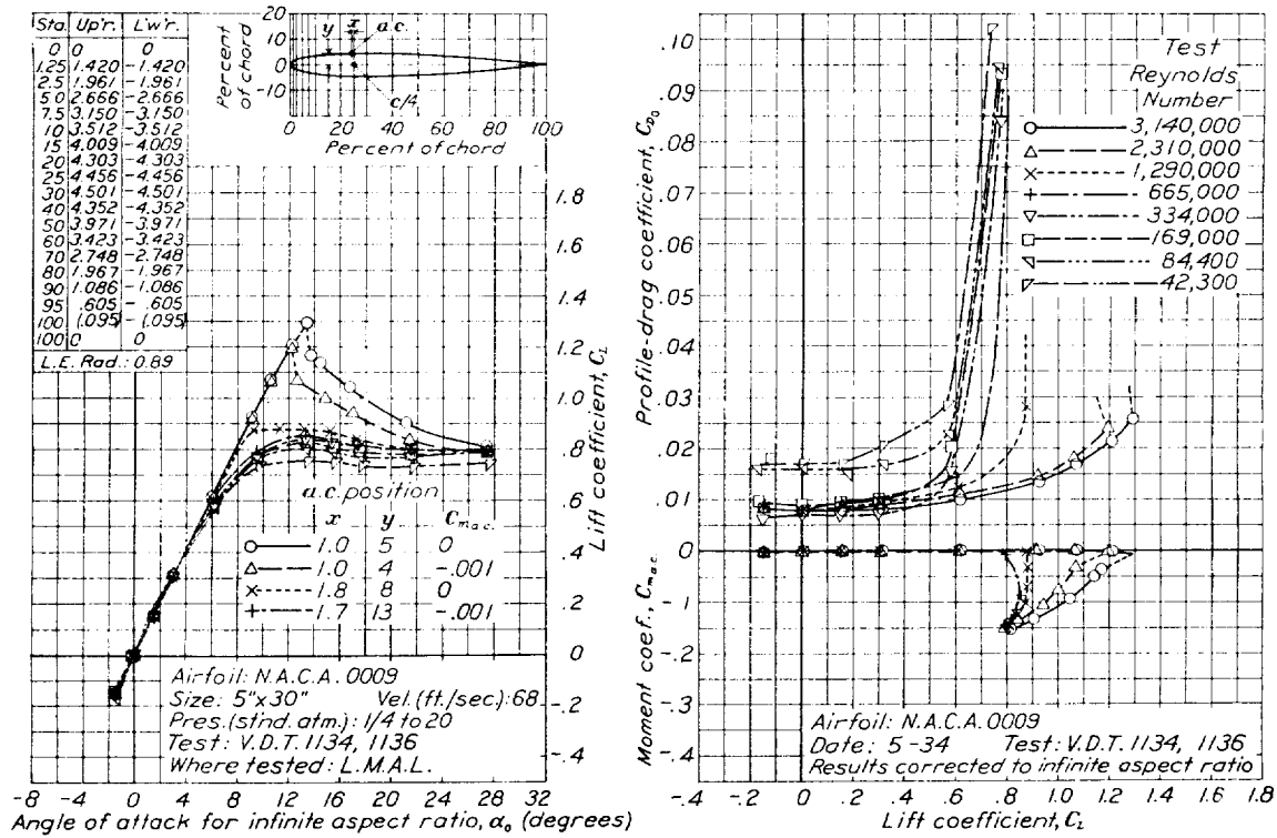
FIGURE 2.—N. A. C. A. 0009.
