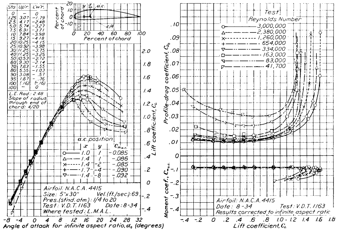
FIGURE 10.—N. A. C. A. 4415.
