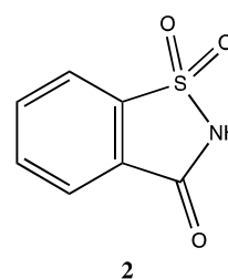
2H-1λ 6 ,2-benzothiazol-1,1,3-trione (Saccharin)
