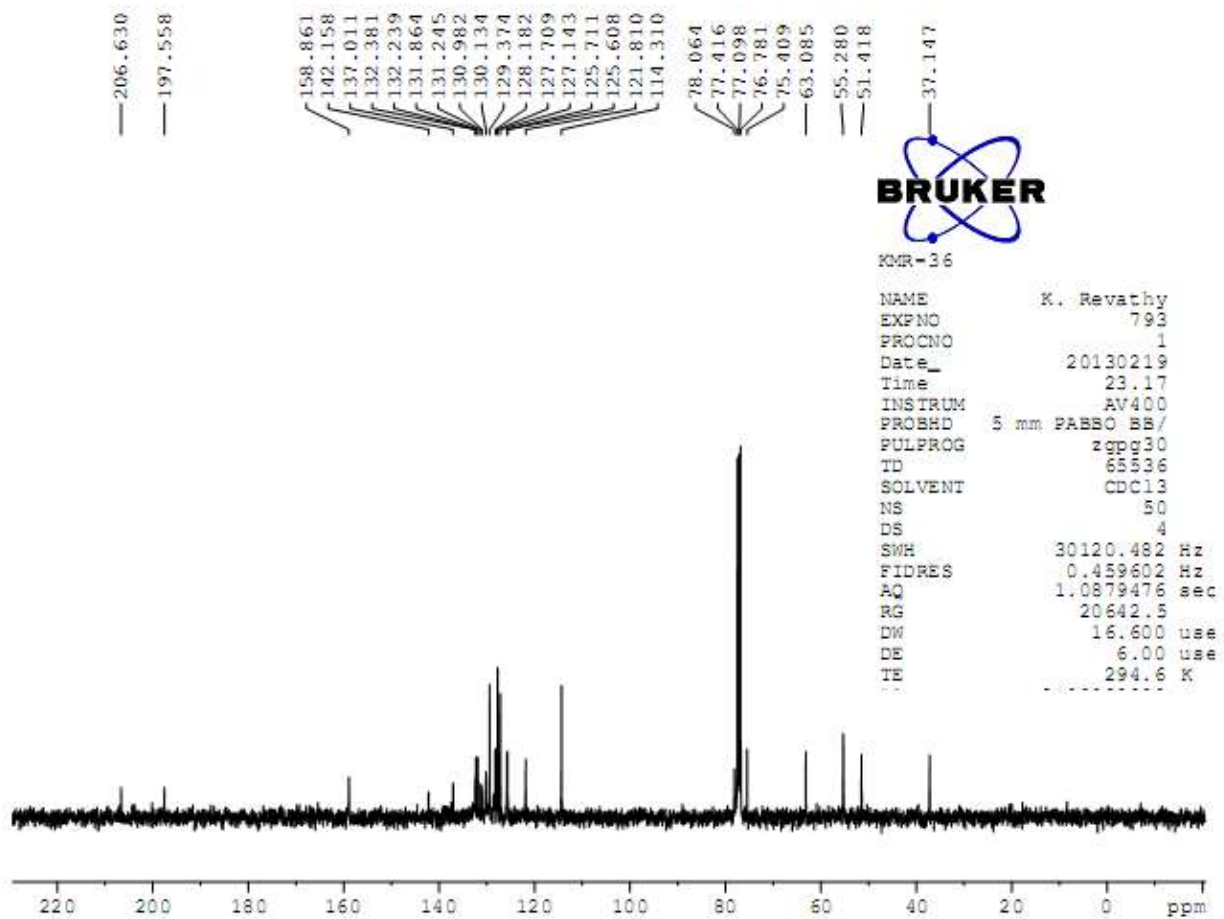
^{13}\text{C} NMR Spectrum of 10e
