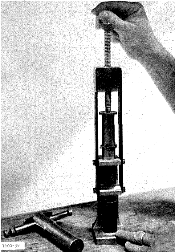
Fig. A-6. Use of Hvorslev technique
