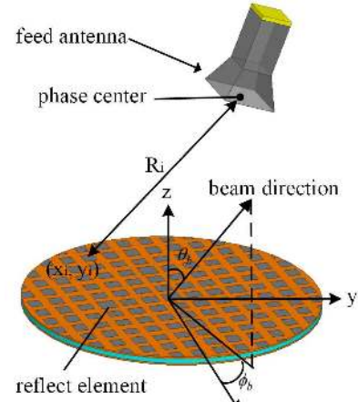
Fig. 1. Configuration of reflectarray antennas.
