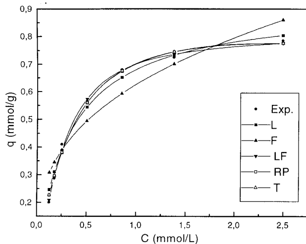
Figura 3. Ajustes dos dados experimentais de adsorção de Cu(II) com QTDH empregando as isotermas de Langmuir (L), Freundlich (F), Langmuir-Freundlich (LF), Redlich-Peterson (RP), Tóth (T).
