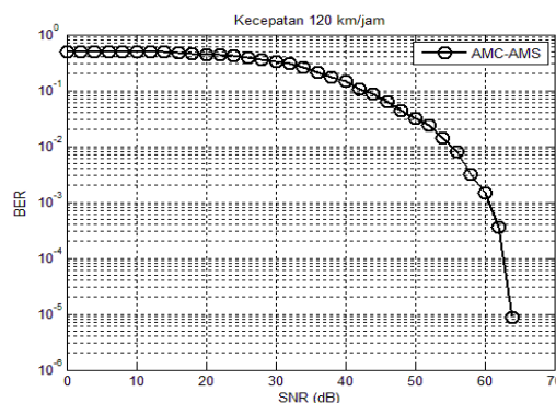
Gambar 7. Grafik BER Terhadap SNR Sistem Dengan Kombinasi Teknik AMC Dan AMS Saat Kecepatan Bergerak Pengguna Sebesar 120 Km/Jam
