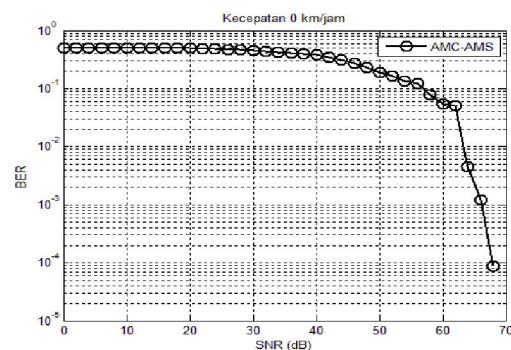
Gambar 6. Grafik BER Terhadap SNR Sistem dengan Kombinasi Teknik AMC dan AMS Saat Kecepatan Bergerak Pengguna Sebesar 0 Km/Jam
