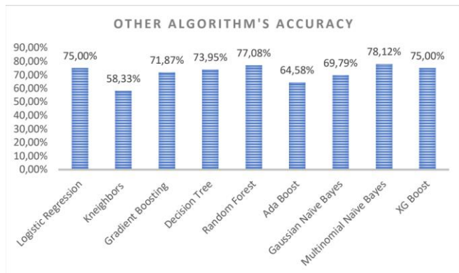
Gambar 7. Grafik Perbandingan Accuracy Algoritma Lain.
