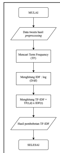
Gambar 4. Alur Proses Pembobotan TF-IDF
