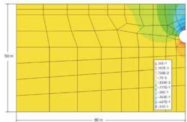
Slika 7. Konture vertikalnih pomaka u poprečnom presjeku y = -50 \text{ m}
