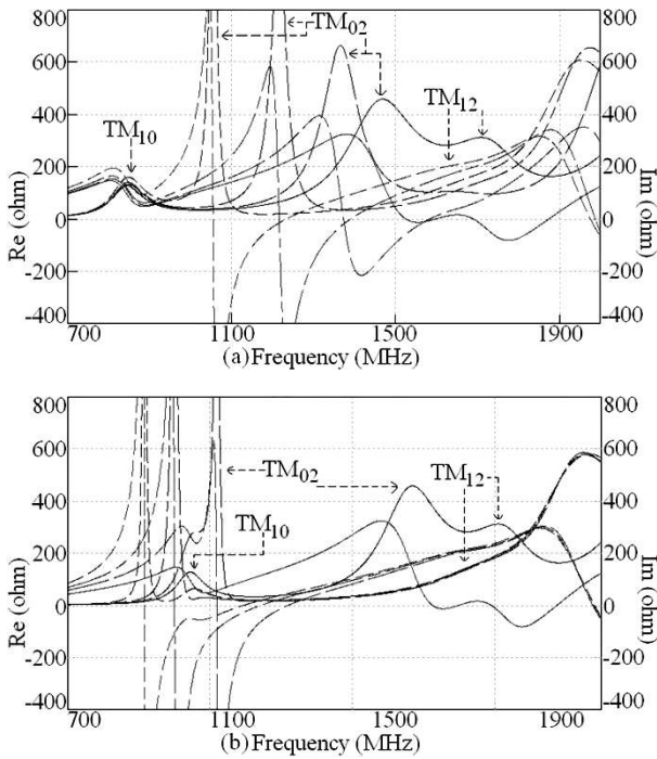
Fig. 6 Resonance curve plots for (a) (—) RMSA, (---) l_s = 2.0 , (---) l_s = 3.0 , (---) l_s = 4.0 , (b) (—) RMSA, (---) l_s = 5.0 , (---) l_s = 6.0 , (---) l_s = 7.0 for E-shaped MSA in 900 MHz frequency range
