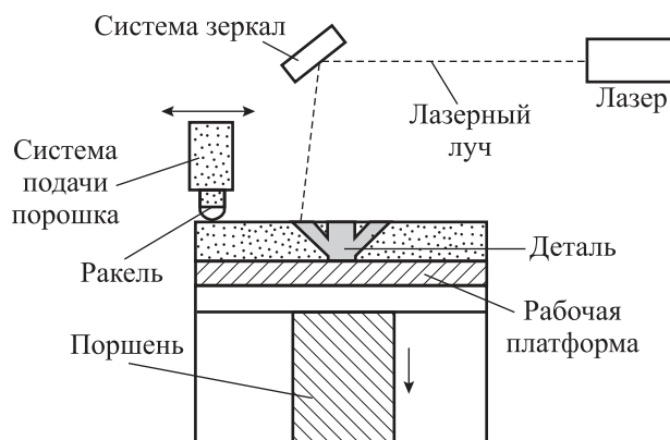
Рис. 1. Принципиальная схема процесса СЛП
