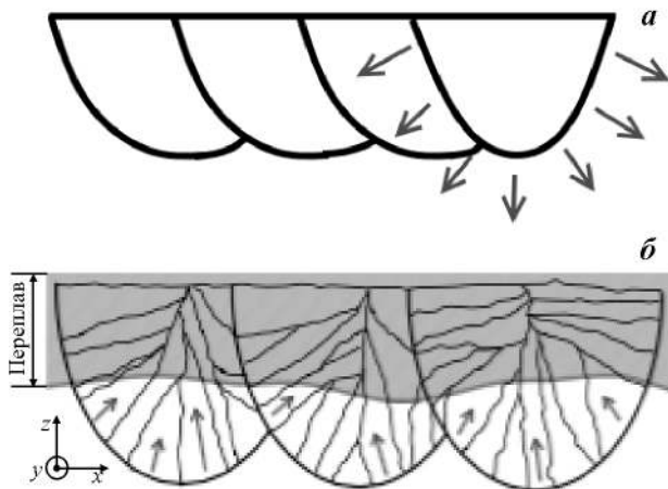
Рис. 5. Схемы теплоотвода в ванне расплава при селективном лазерном плавлении (а) и переплава нижележащего слоя (б) [9]
