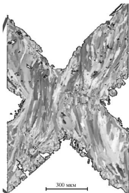
Рис. 7. Изображение зеренной структуры сетчатой конструкции, полученное дифракцией отраженных электронов [28]
