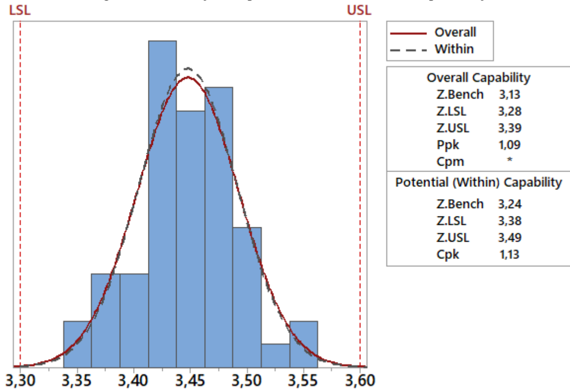
Figura 17 – Variação do peso dentro dos limites de especificação
