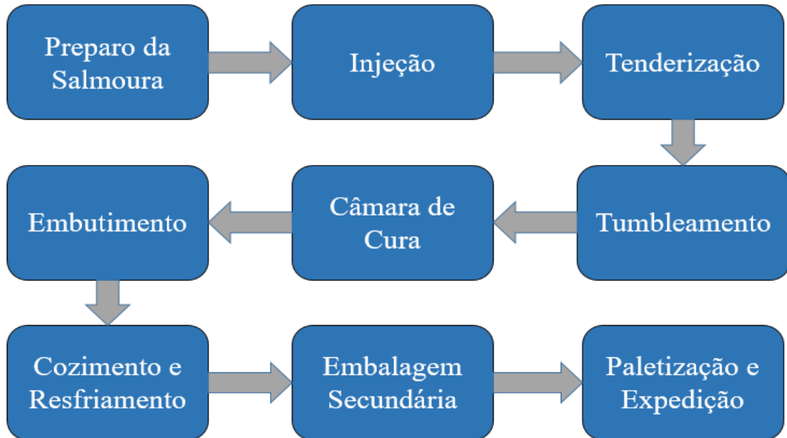
Figura 8 – Fluxograma do processo produtivo do presunto
