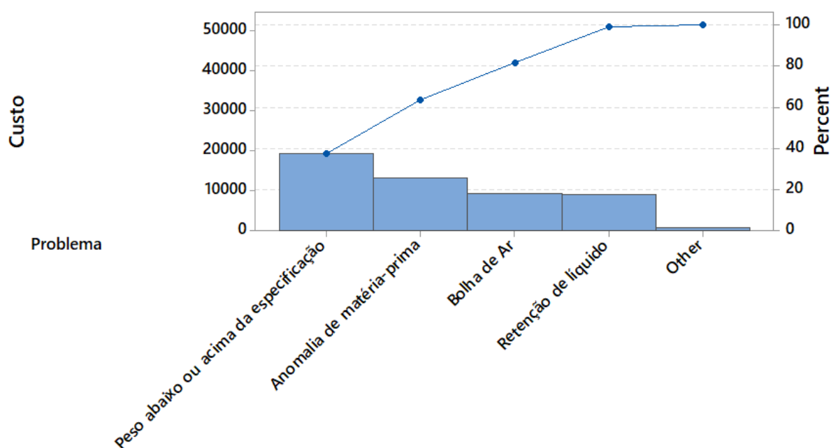
Figura 9 – Gráfico de Pareto para os problemas
