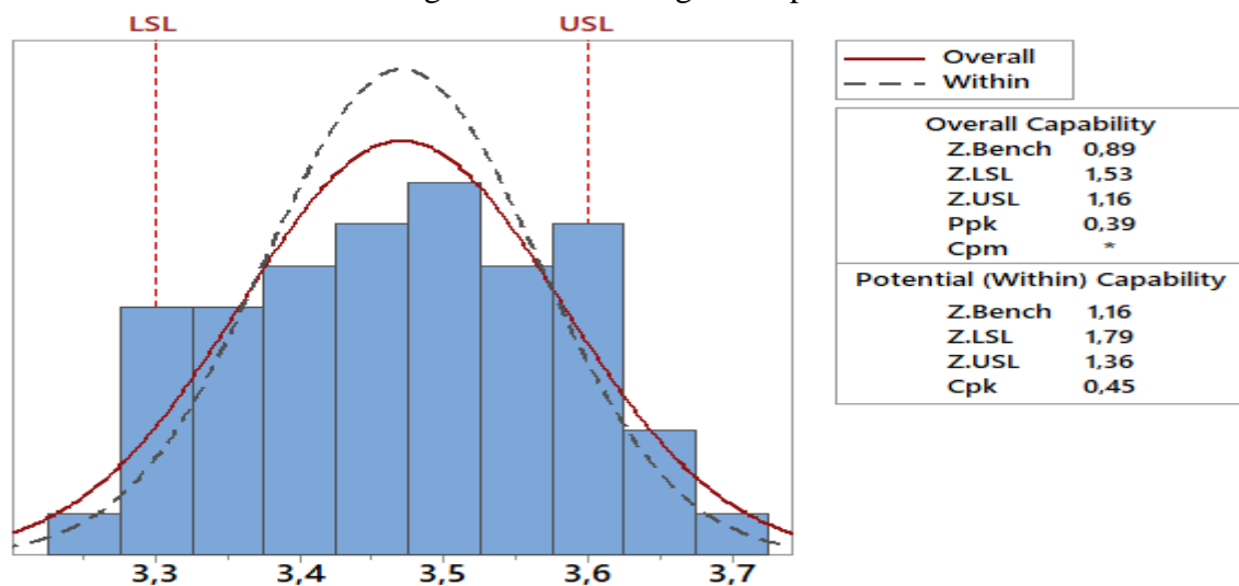
Figura 12 – Nível sigma do processo
