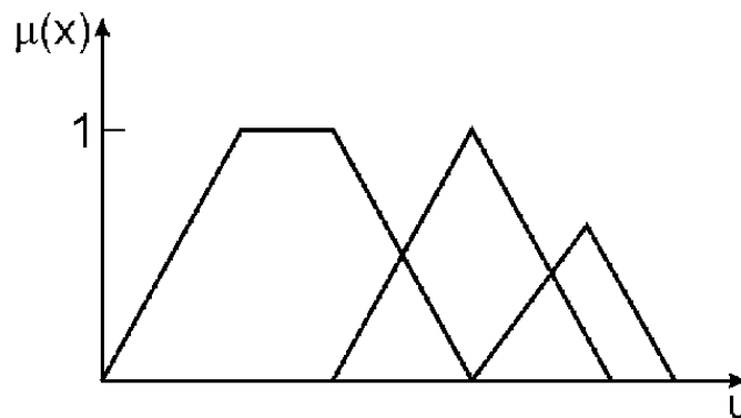
Figura 2.2: Exemplo de função de pertinência do tipo linear por partes.
