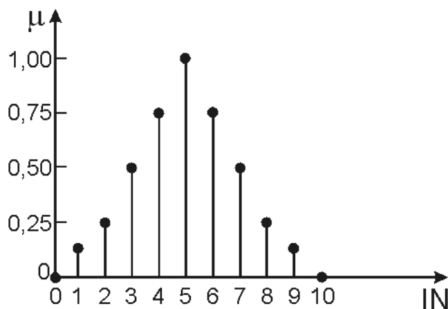
Figura 1.1: Função de pertinência do conjunto fuzzy que corresponde aos números aproximadamente iguais a 5 , no universo dos \mathbb{N} .
