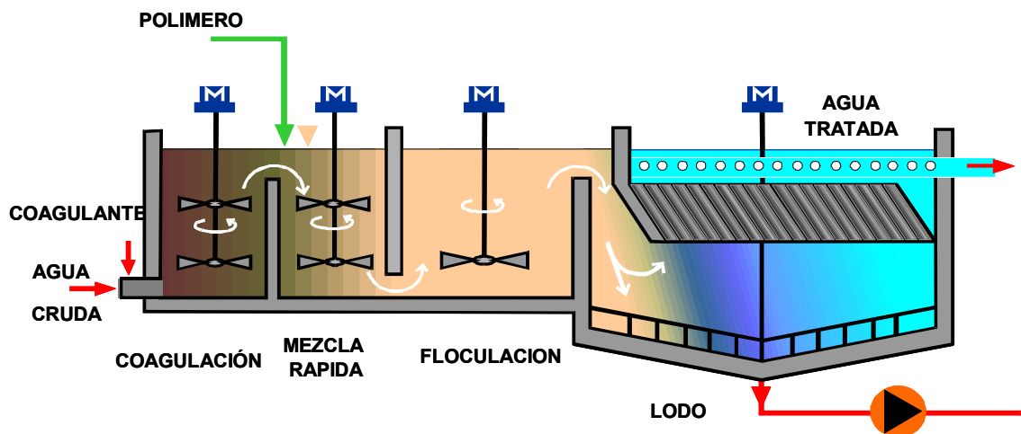
Figura 1. Esquema típico de Coagulación / Floculación / Sedimentación.
