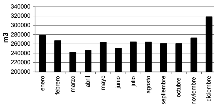
Figura 5. Volúmenes medios mensuales de agua distribuida (Período 2000-2003).
