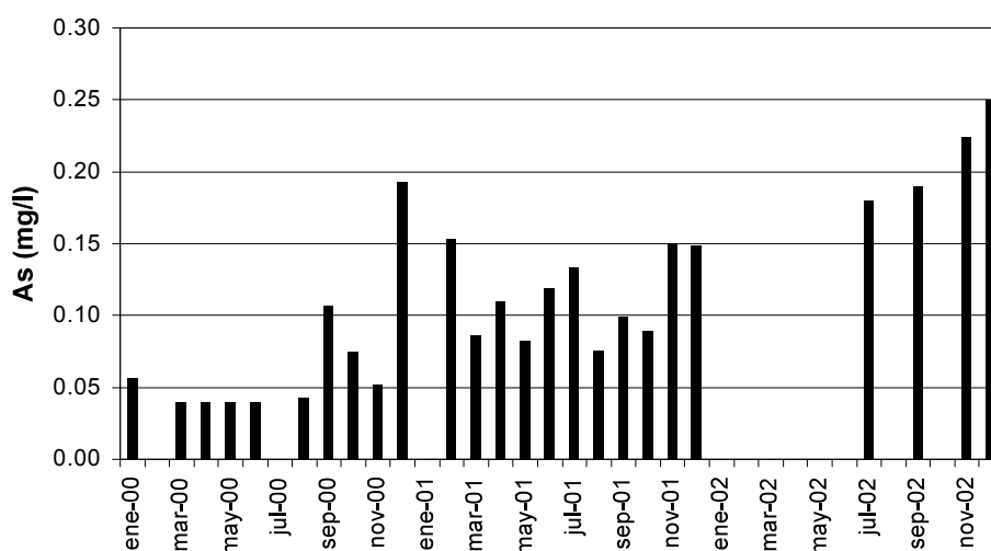
Figura 4. Evolución temporal de los niveles de arsénico en el pozo N° 18.
