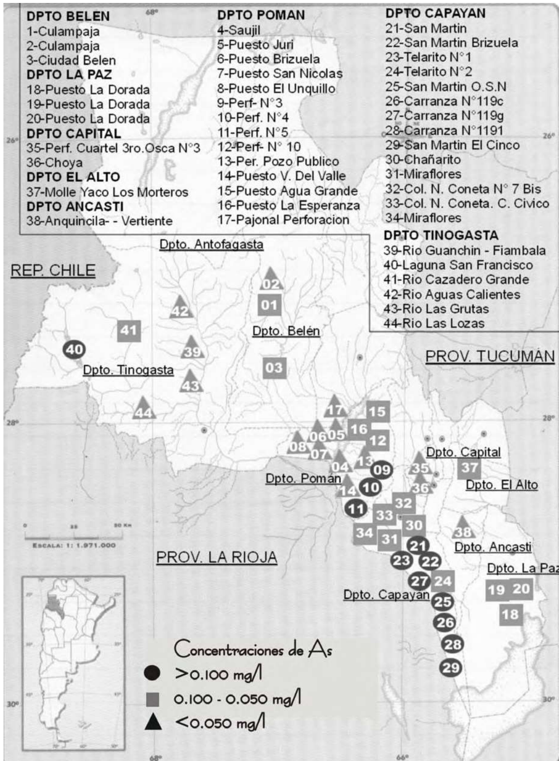
Figura 1. Distribución de las concentraciones de arsénico en la provincia de Catamarca. República Argentina. Los números corresponden a los listados de lugares de la parte superior del mapa. Los símbolos indican concentraciones de arsénico.
