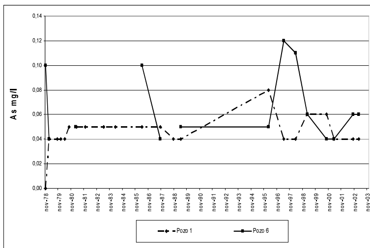
Figura 4. Evolución en el contenido de As en Realicó.
