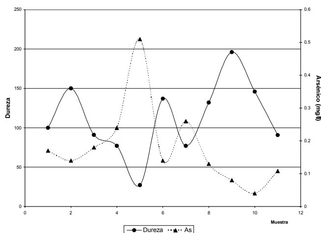
Figura 4. Correlación As – Dureza del agua en cada una de las muestras.
