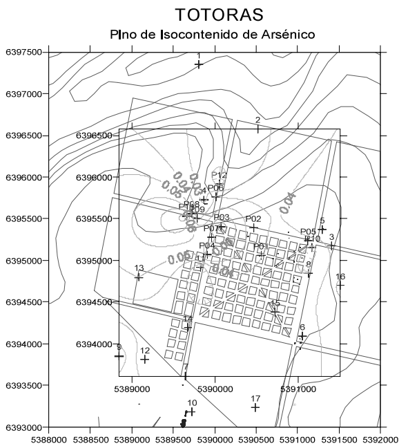
Figura 4. Plano de isocontenidos de As.
