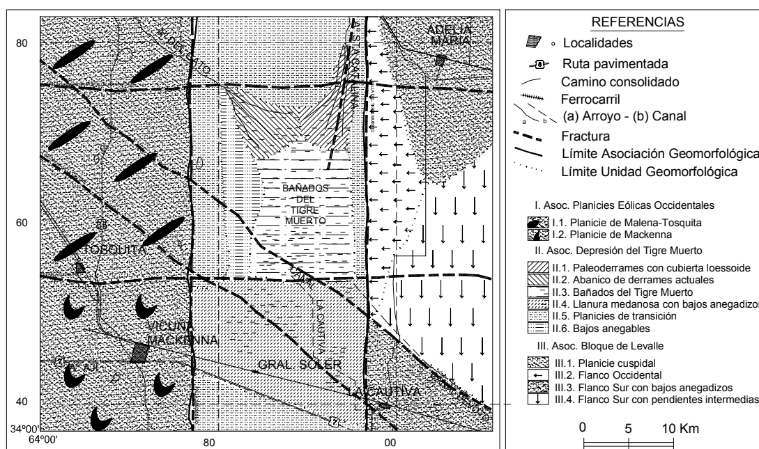
Figura 2. Mapa geológico-geomorfológico. Tomado de Villalba et al. (2002).
