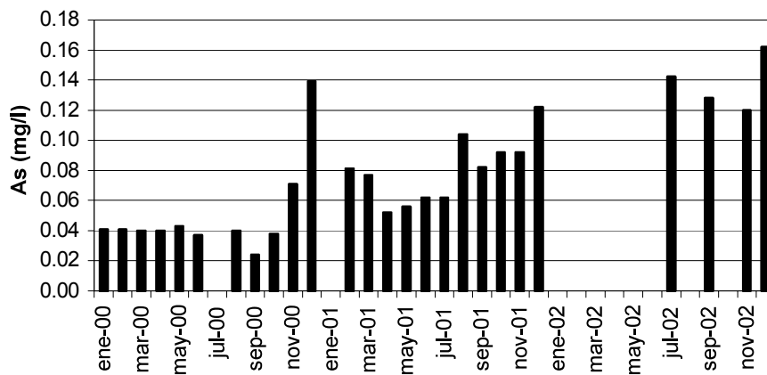
Figura 3. Evolución temporal de los niveles de arsénico en el pozo N° 24.
