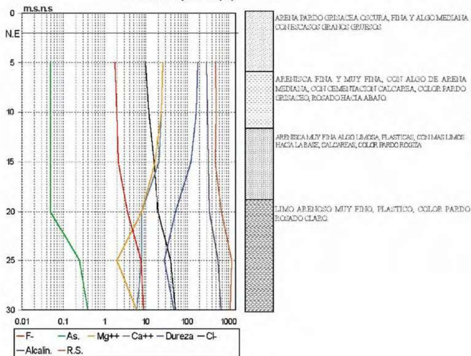
Figura 6. Evolución hidroquímica en profundidad para Anguil (valores expresados en mg/l).
