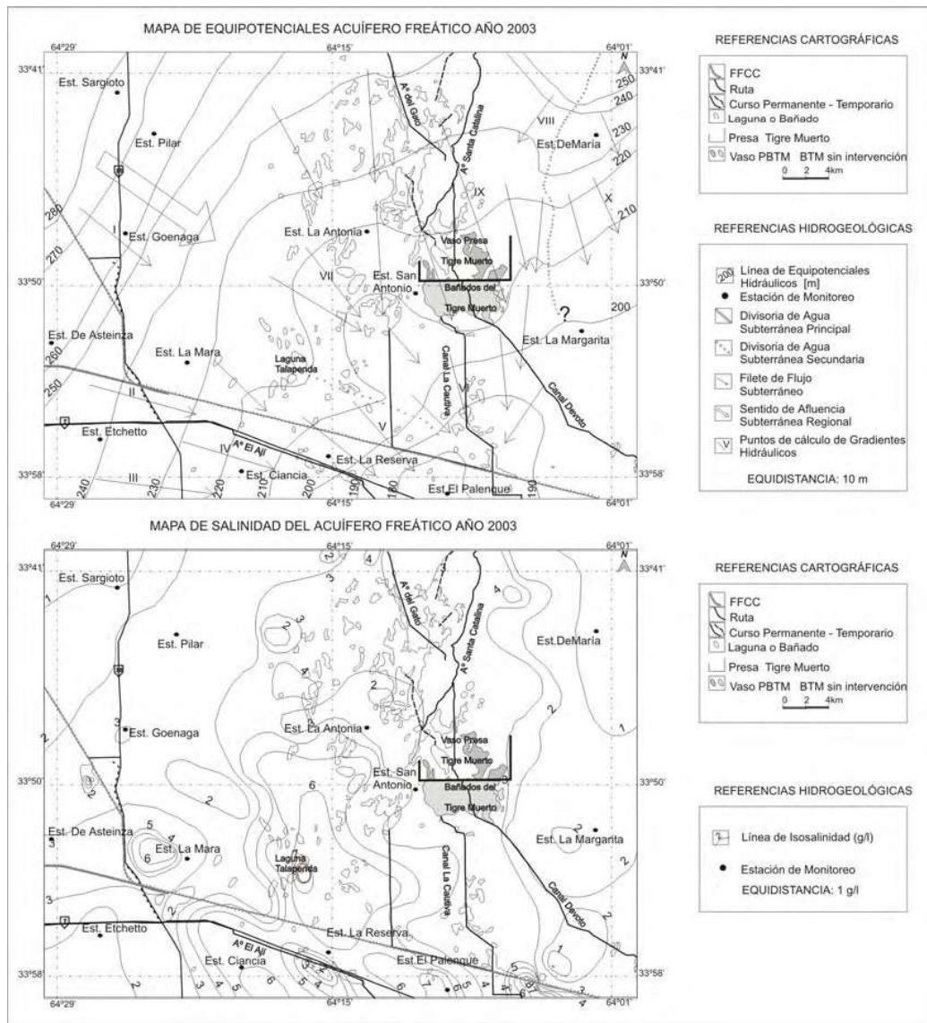
Figura 3. Mapa de potenciales hidráulicos y de salinidad del acuífero libre.
