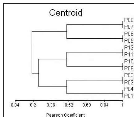
Figura 7. Análisis de cluster.
