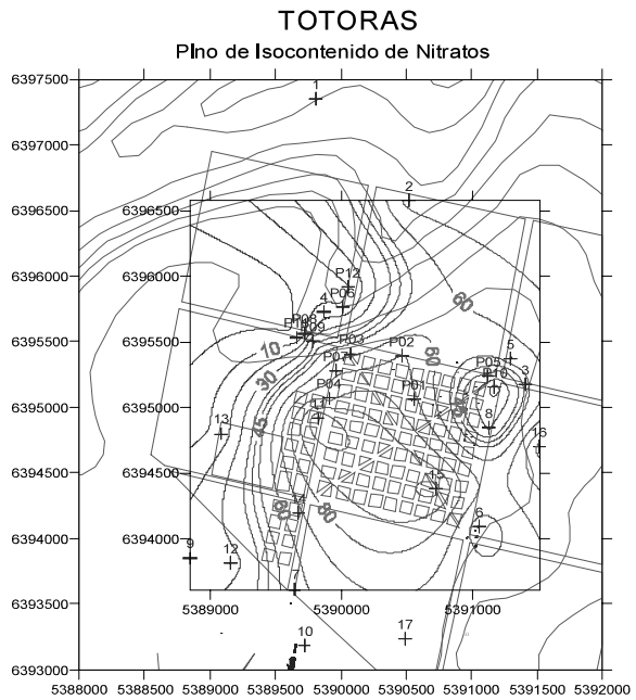
Figura 5. Plano de isocontenidos de NO 3 .
