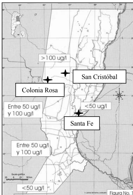
Figura 1. Concentraciones de arsénico y plano de ubicación.
