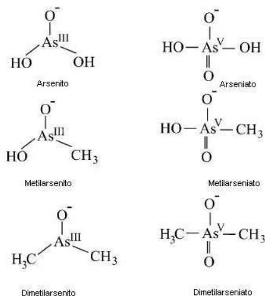
Figura 1. Especies de arsénico encontradas en el agua.
