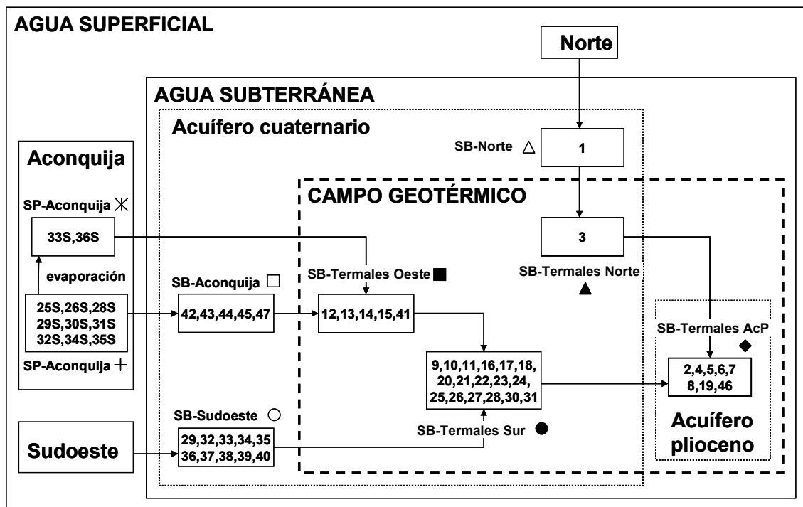
Figura 3. Modelo conceptual de las relaciones entre aguas superficiales y subterráneas atermales y termales.
