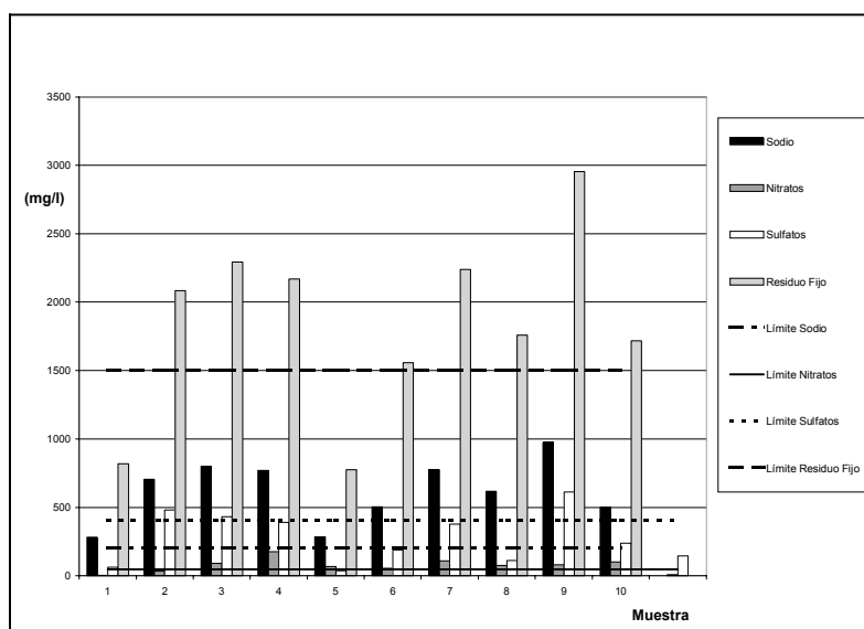
Figura 3. Parámetros fisicoquímicos analizados y situación en cada una de las muestras respecto a la Ley Provincial N° 11.220.
