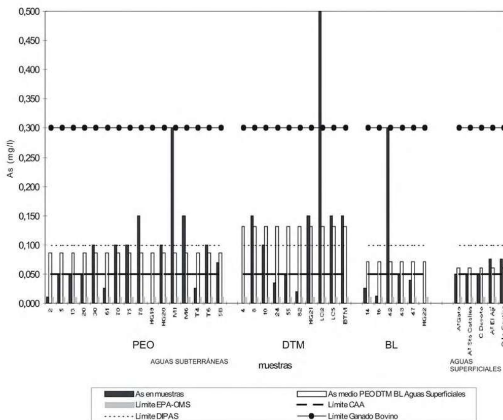
Figura 4. As en aguas superficiales y subterráneas.
