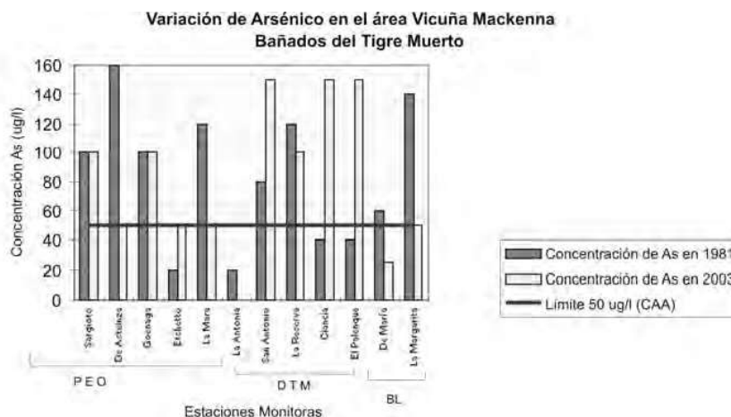
Figura 7. As en aguas subterráneas en los años 1981 y 2003.
