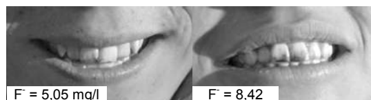
Figura 8. Evidencias de fluorosis dental en adolescentes y tenores de F - del agua subterránea que consumen. Malena
