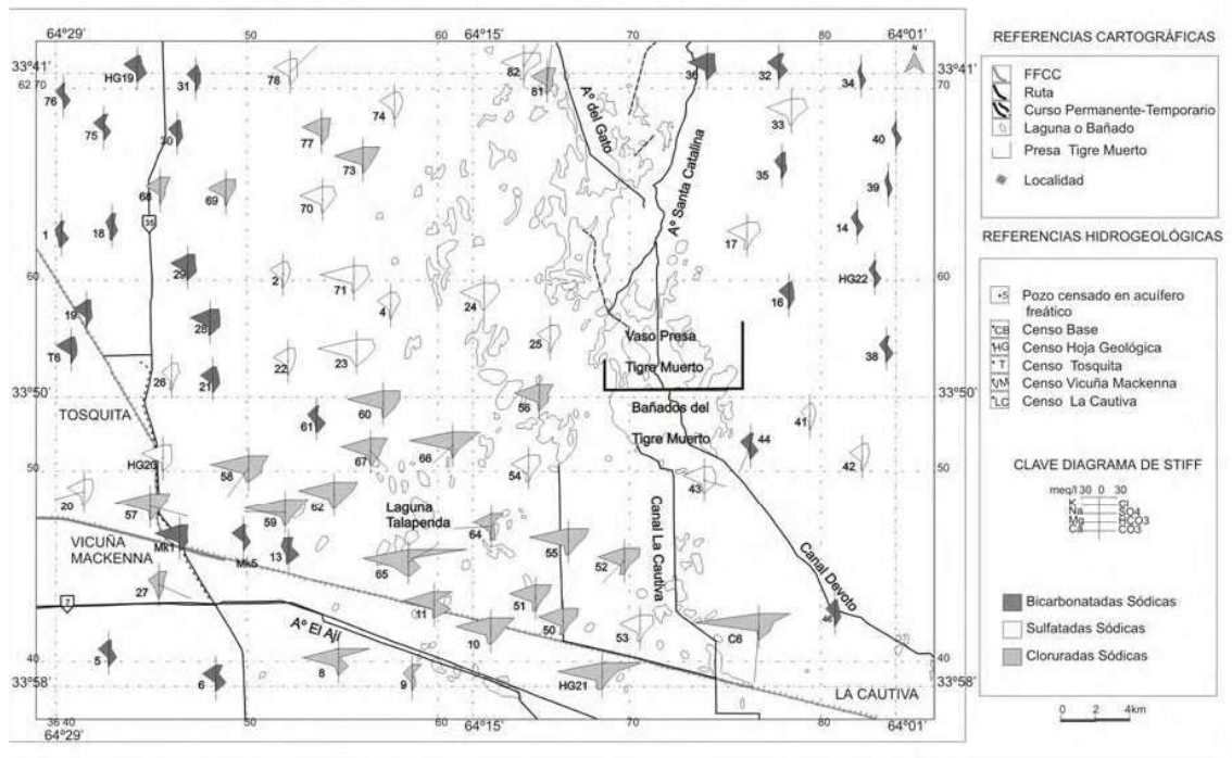
MAPA CON DIAGRAMAS DE STIFF ACUÍFERO LIBRE AÑO 2003
