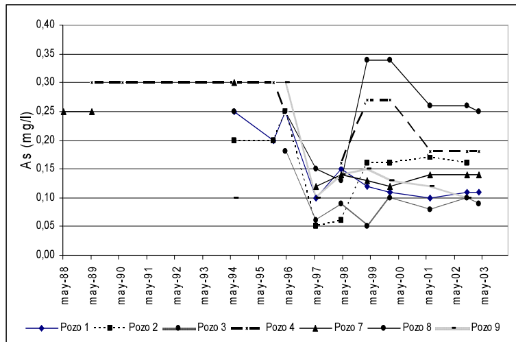
Figura 3. Evolución en el contenido de As en Eduardo Castex.
