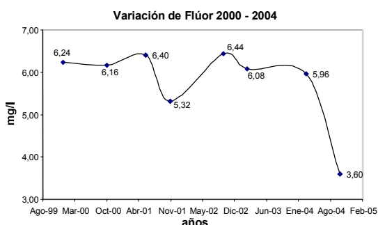
Fig. 1. Variación de la concentración de Fluor entre los años 2000 – 2004.
