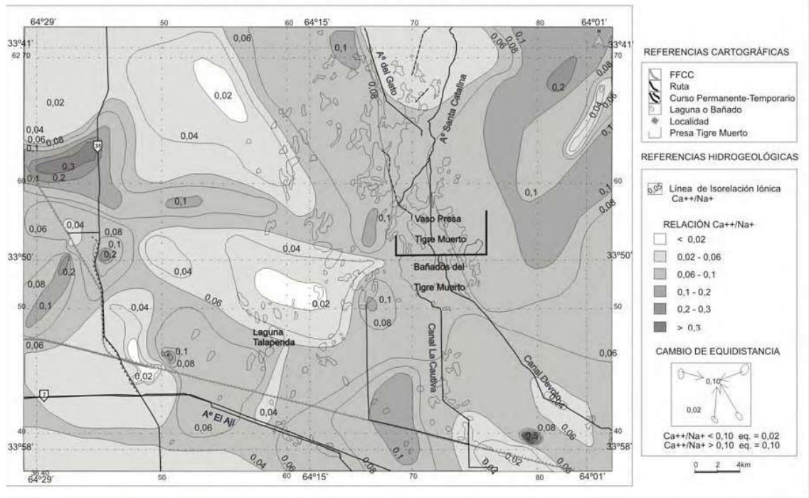
MAPA DE RELACIÓN IÓNICA Ca ++ /Na + ACUÍFERO LIBRE AÑO 2003
