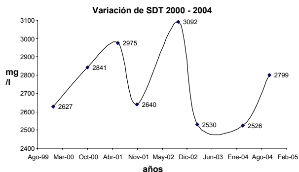
Fig. 3. Variación de la concentración de Sólidos Disueltos Totales entre los años 2000 – 2004.
