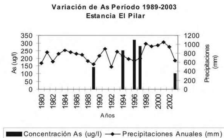
Figura 8. Variación As en aguas subterráneas en los años 1989 a 2003.
