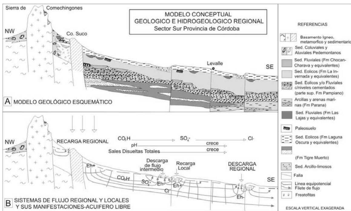
Figura 2. Perfil geológico e hidrogeológico regional.
