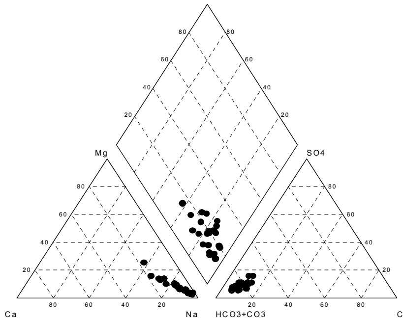
Figura 2. Diagrama de Piper de las aguas subterráneas.
