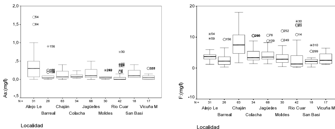
Figura 6. Diagrama de Cajas para As y F -
