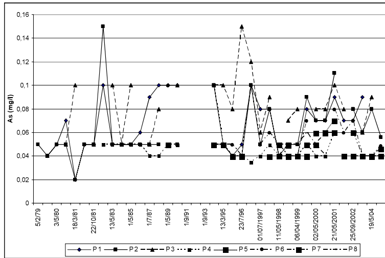
Figura 2. Evolución en el contenido de As en Macachín.
