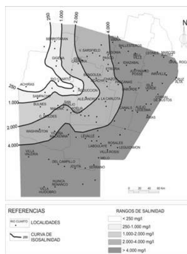
Figura 4. Mapa de salinidad. Acuífero freático. Sur de Córdoba.
