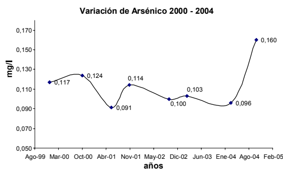
Fig. 2. Variación de la concentración de arsénico entre los años 2000 – 2004.
