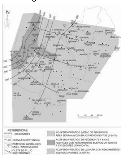
Figura 3. Mapa equipotencial. Acuífero freático. Sur de Córdoba.
