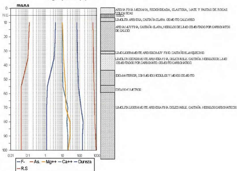
Figura 5. Evolución hidroquímica en profundidad para Anchorena (valores expresados en mg/l).
