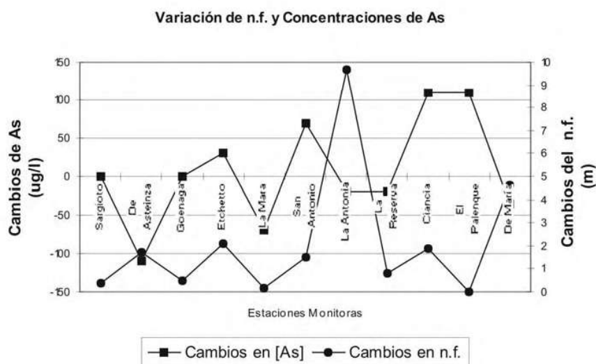
Figura 9. Variación de As y niveles freáticos en los años 1981 y 2003.
