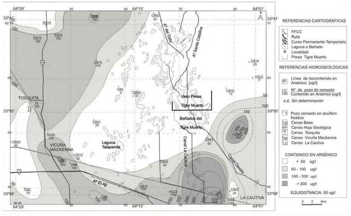
MAPA DE DISTRIBUCIÓN DE ARSÉNICO ACUÍFERO LIBRE AÑO 2003
