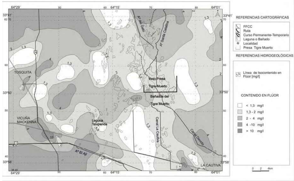
MAPA DE DISTRIBUCIÓN DE FLÚOR ACUÍFERO LIBRE AÑO 2003
