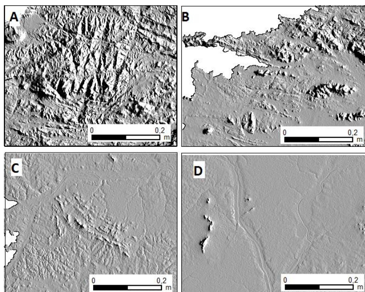
Figura 5. Padrões morfológicos de sistemas denudacionais e agradacionais. (A) – região do Complexo Parima-Pacaraima, forte dissecação e controle estrutural ( 4^{\circ}62'N 60^{\circ}67'W ); (B) –, Transição entre lavrado e floresta ombrófila, município de Pacaraima, com forte dissecação e controle estrutural ( 4^{\circ}29'N 60^{\circ}33'W ); (C) – rio Uaricoera, dissecação moderada dissecação média, com controle estrutural, transição de morfologias agradacionais e denudacionais ( 3^{\circ}30'N 61^{\circ}33'W ); (D) – Confluência dos rio Tacutu e Uaricoera, com predominância de morfologias agradacionais ( 3^{\circ}12'N 60^{\circ}29'W ).
