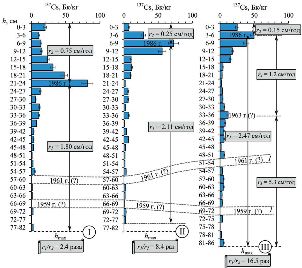
Рис. 4. Распределение концентрации радиоизотопа ^{137}\text{Cs} по глубине ( h ) в почвенных (стратоземы) разрезах I, II и III (см. рис. 3) дна изученного участка Куреговской балки, Удмуртская Республика
