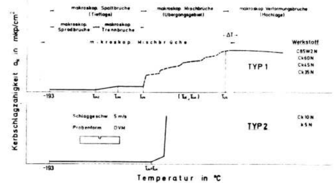
Schematischer Verlauf von Kerbschlagzähigkeits-Temperatur-Kurven und Brucharten
