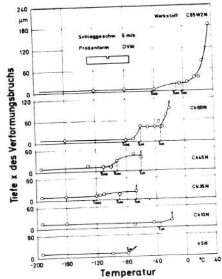
Mikrofraktographische Analyse des Bruchverhaltens von Kerbschlagbiegeproben im Kerngrund im Splitbruchgebiet
